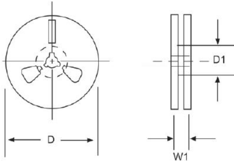
Fig 4. Reel dimensions
